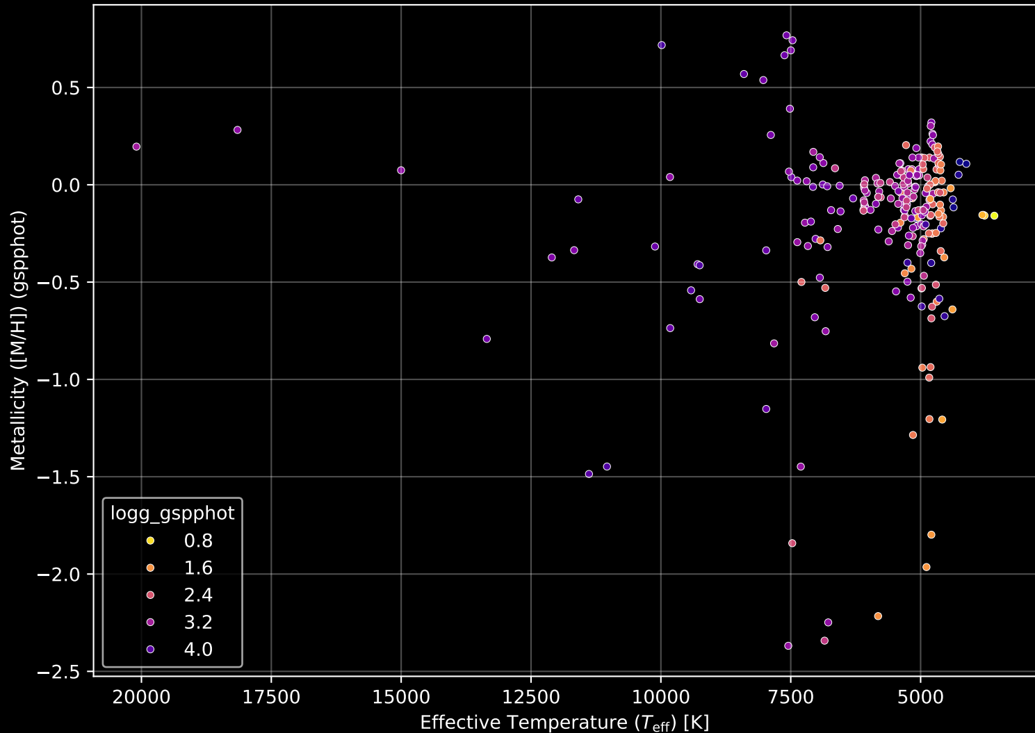
APOGEE DR17 Field: [Berkeley_2_btx] Stellar Population Parameters (n= 252)
